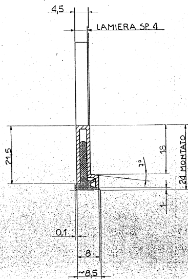
SEZIONE PARZIALE A-A SCALA 2:1
