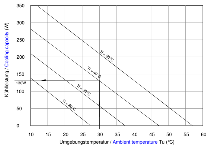
Leistungsdiagramm / Performance curve PK 50
